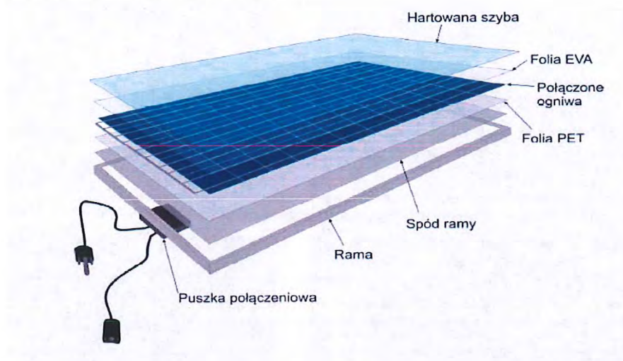
Rysunek 21. Budowa modułu fotowoltaicznego
